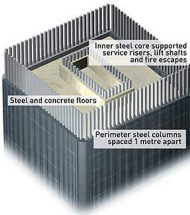
Техническая схема башен-близнецов
