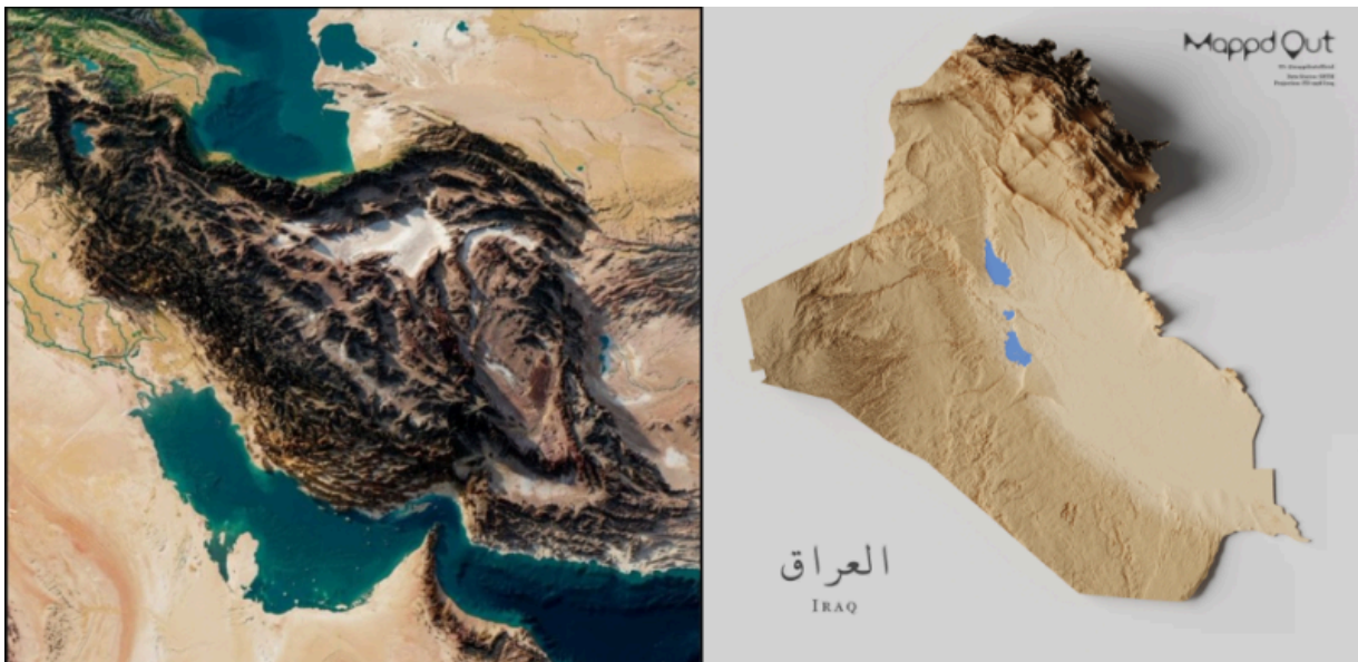
Topographische Karten des Irans (links) und des Iraks (rechts)
